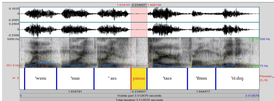
Рисунок 1 Осциллограмма, спектрограмма, графики ЧОТ и интенсивности, транскрипция и сегментация на уровне фонетических слов синтагмы When my eyes tire from reading в реализации диктора – носителя японского языка
