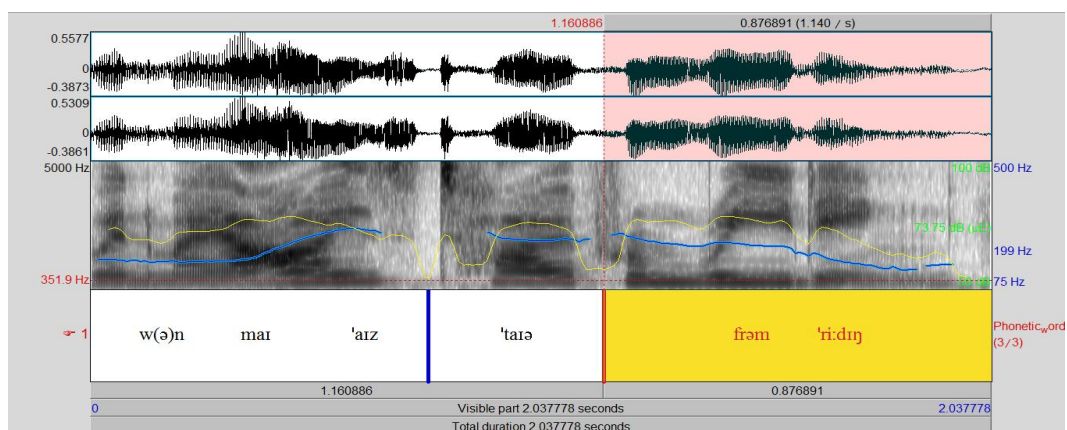
Рисунок 4 Осциллограмма, спектрограмма, графики ЧОТ и интенсивности, транскрипция и сегментация на уровне фонетических слов синтагмы When my eyes tire from reading в реализации диктора – американца
