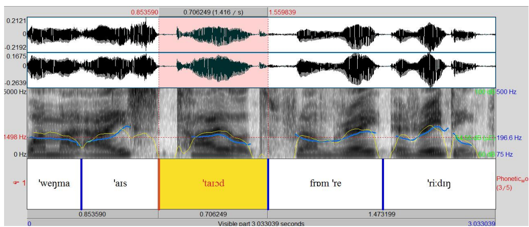
Рисунок 3 Осциллограмма, спектрограмма, графики ЧОТ и интенсивности, транскрипция и сегментация на уровне фонетических слов синтагмы When my eyes tire from reading в реализации диктора – носителя китайского языка
