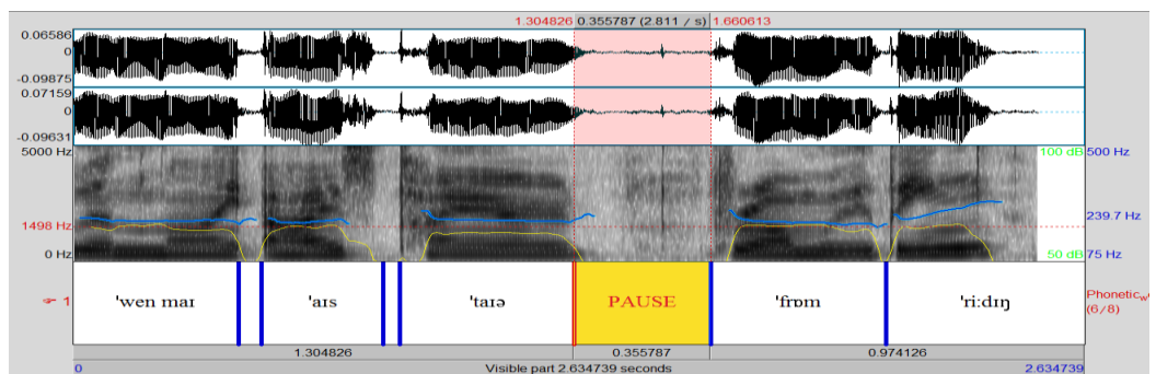
Рисунок 2 Осциллограмма, спектрограмма, графики ЧОТ и интенсивности, транскрипция и сегментация на уровне фонетических слов синтагмы When my eyes tire from reading в реализации диктора – носителя корейского языка
